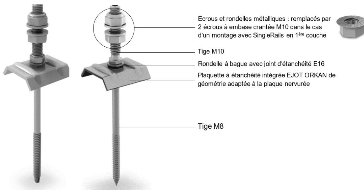
Vis de fixation pour panneaux solaires : (gauche) pour pannes en acier ; (droite) pour pannes en bois
