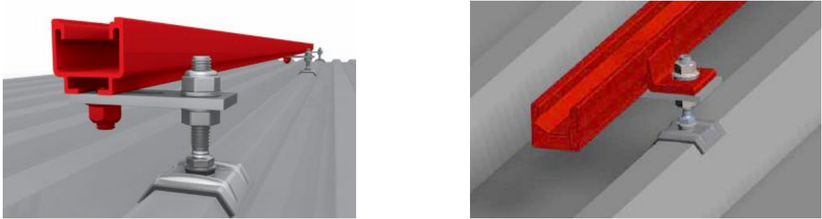
Illustrations de l'assemblage {vis de fixation panneaux solaires + adaptateur + rail 1 ère couche} Gauche : 1 ère couche = SolidRail. Droite : 1 ère couche = SingleRail.
