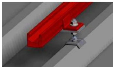
Cas du montage avec SingleRails en 1 ère couche
