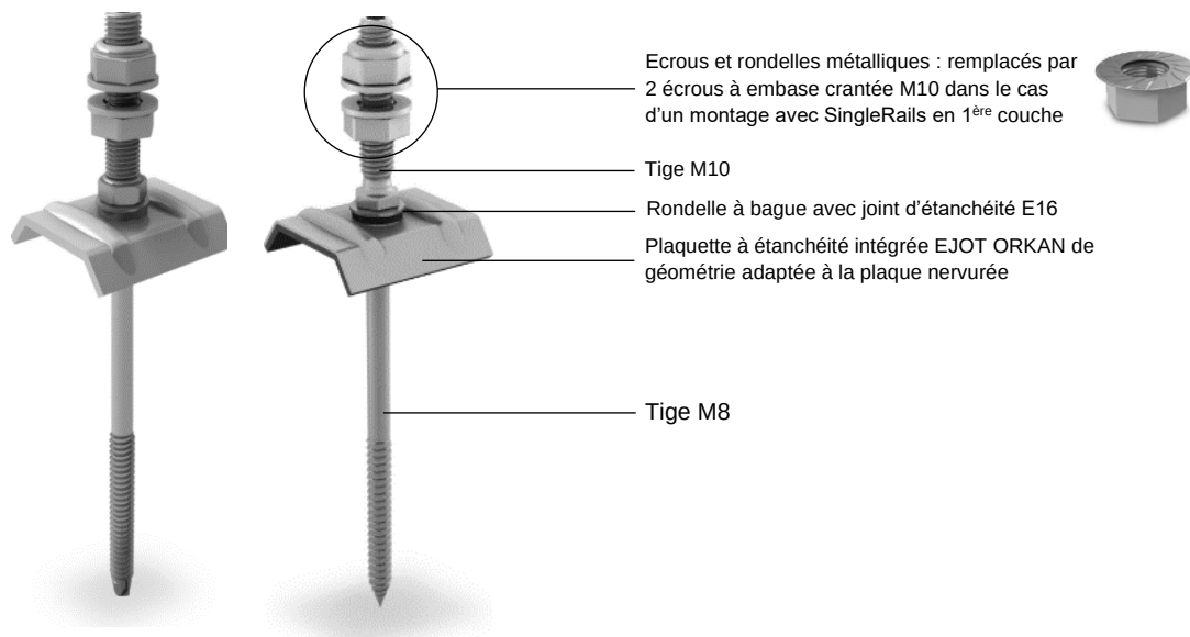
Vis de fixation pour panneaux solaires : (gauche) pour pannes acier ; (droite) pour pannes bois
