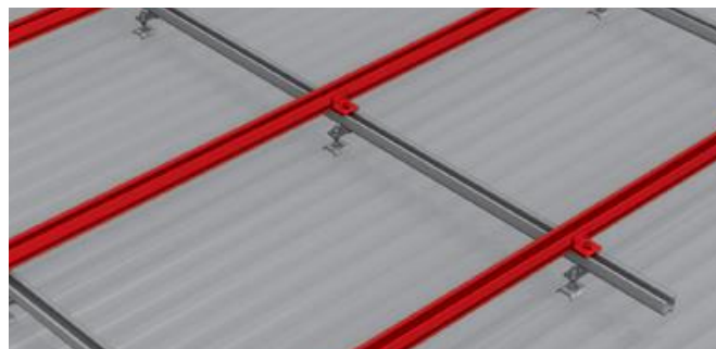
Illustration du procédé K2 SOLARFASTENER PLAQUES NERVURÉES (DROM) (cas de la configuration B)
