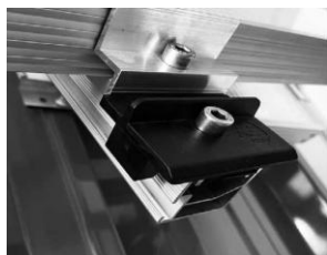
Dispositif anti-glissement pour étrier final standard
