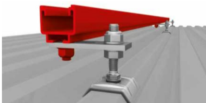
Cas du montage avec SolidRails en 1 ère couche
